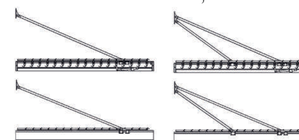
PergoLux oldalnézet normál függesztéssel
