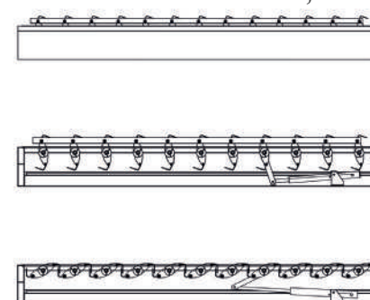
Oldalnézet PergoLux Without oszloppal
