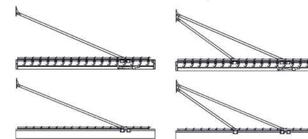
PergoLux oldalnézet normál függesztéssel
