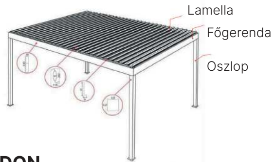
Általános műszaki rajz
