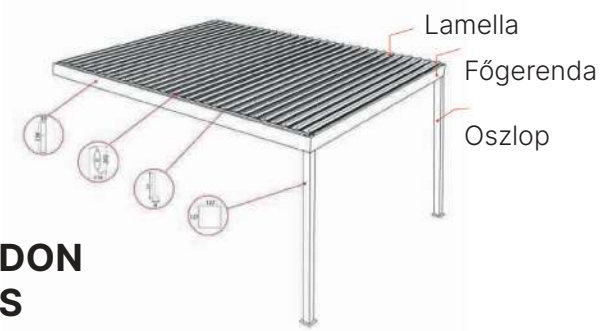
Általános műszaki rajz
