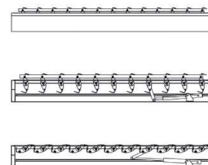
Oldalnézet PergoLux Without oszloppal
